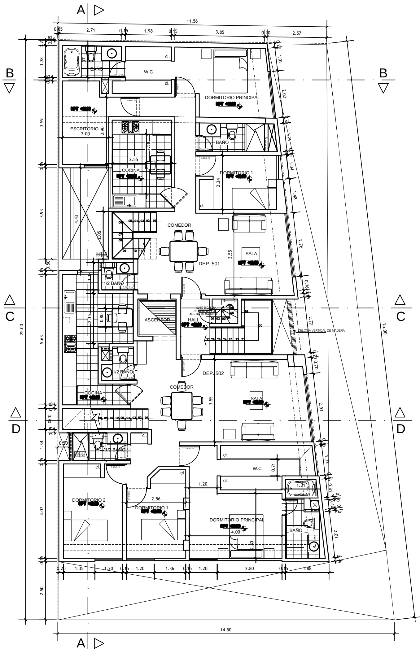
QUINTO PISO
